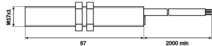
Рис.1. Габаритные размеры излучателя МикРА Ф5И и приемника МикРА Ф5П
