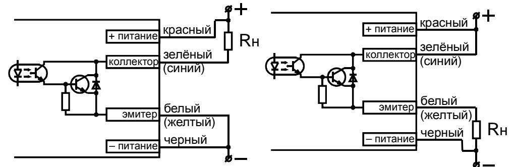
Рис.2. Схемы подключения приемника МикРА Ф5П.
